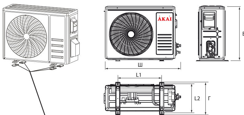
Установка 4 резиновых прокладок (Дополнительно)
