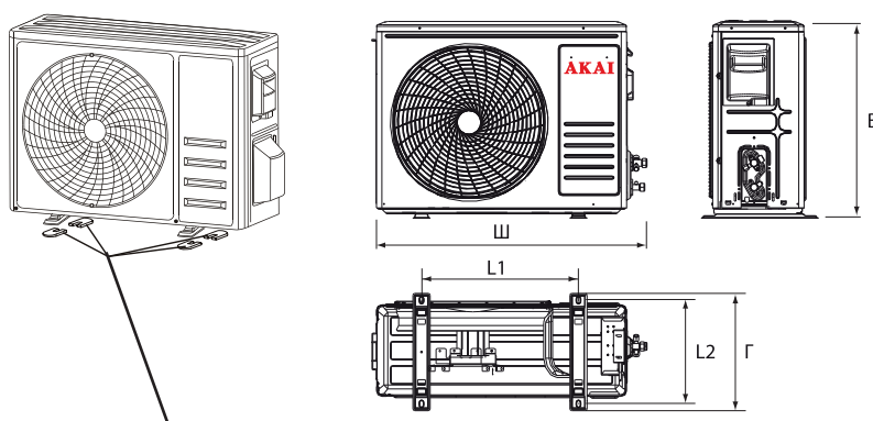
Установка 4 резиновых прокладок (Дополнительно)
